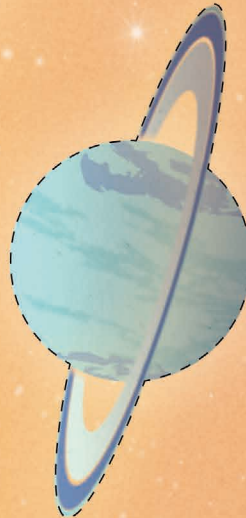
Uranus أورانوس
