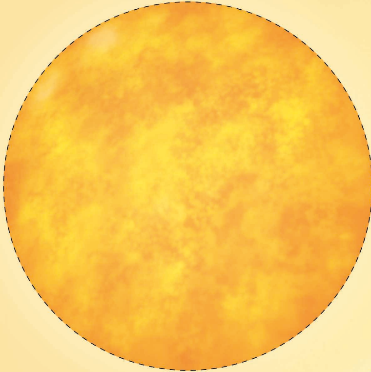
Sonne الشمس
