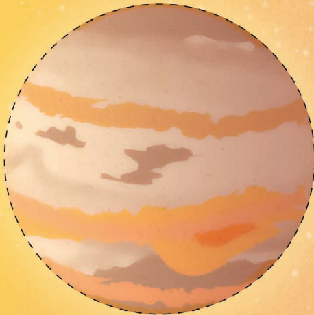
Jupiter المشتري
