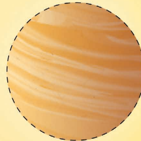
Venus الزهرة
