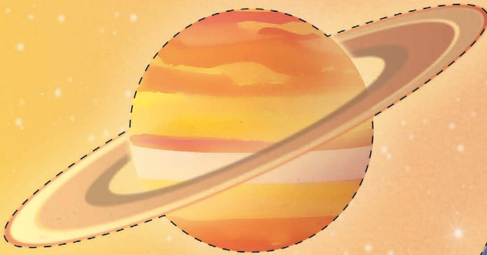
Saturn زحل
