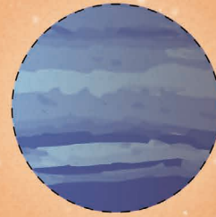
Neptun نبتون
